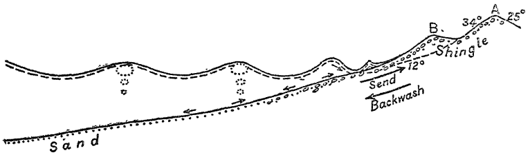
चित्र १२६—तरंगों के टूटने के पहने और बाद जल के कर्णों की गति और बालूतट कगारों का निर्माण।
